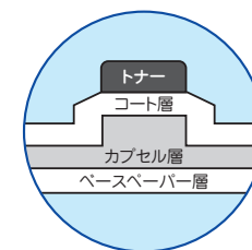
立体コピー断面図
