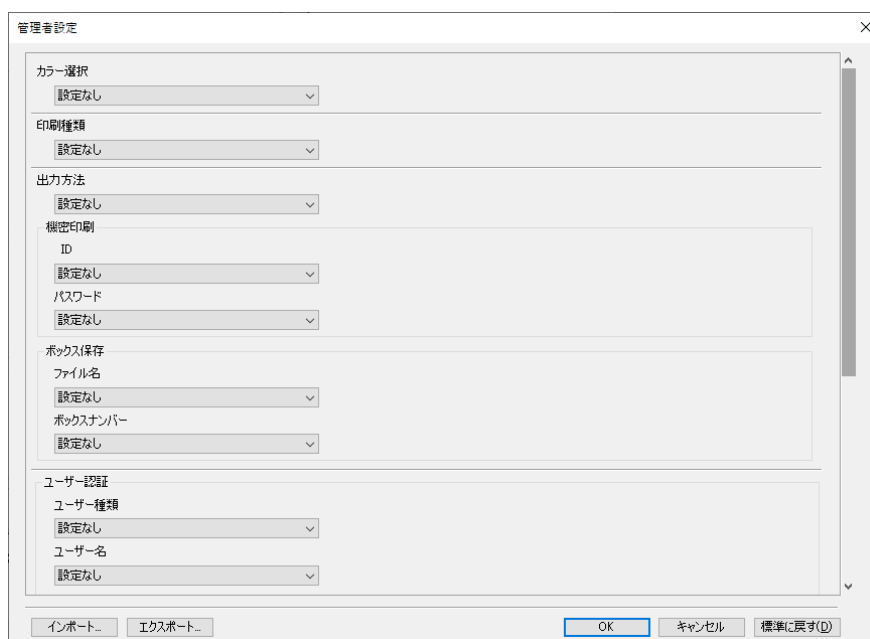
図 4-6-2 管理者カスタマイズ設定画面 1
