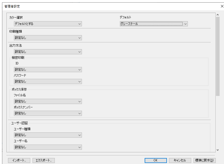
図 4-6-4 管理者カスタマイズ設定画面 3
