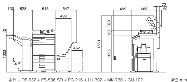
本体 + DF-632 + FS-536 SD + PC-216 + LU-302 + MK-730 + CU-102
